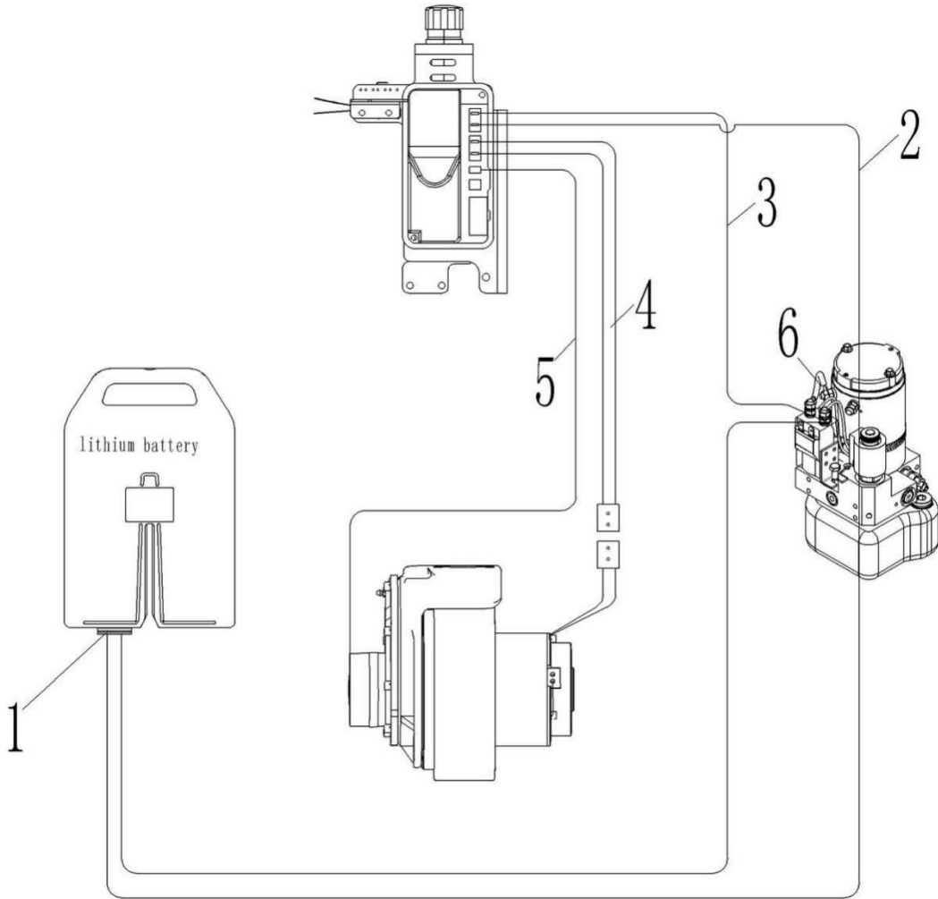
Fig. 18 Wiring Harness
